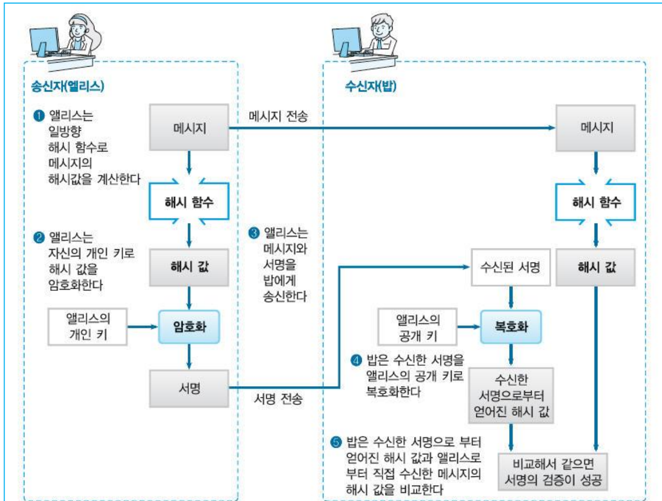
그림 10-6 · 앨리스가 메시지의 해시 값에 서명하고 밥이 서명을 검증한다
