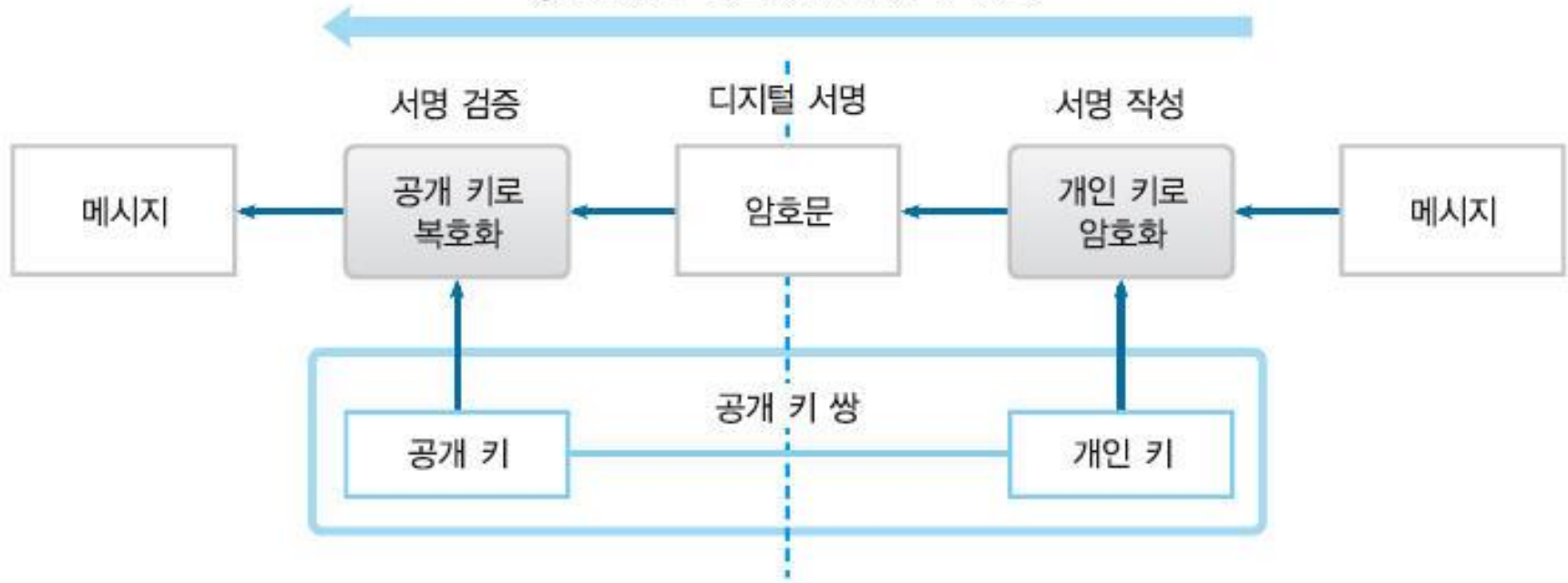
그림 10-2 · 개인 키에 의한 암호화(디지털 서명)
