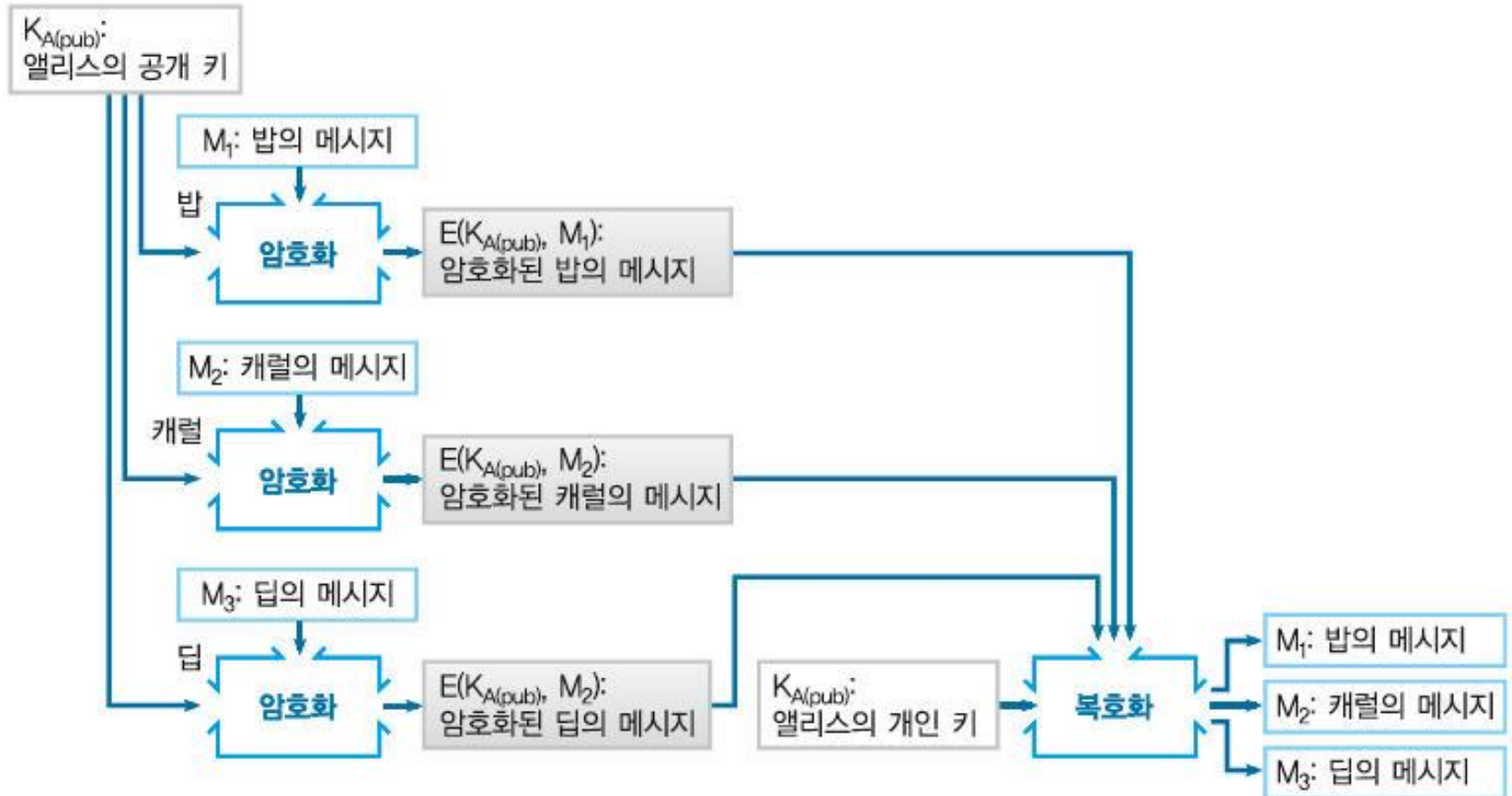
그림 10-3 · 공개 키 암호는 누구라도 암호화할 수 있다(공개 키 암호)
