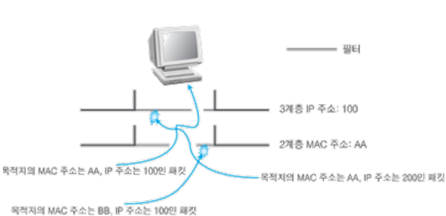
정상적인 네트워크 필터링
