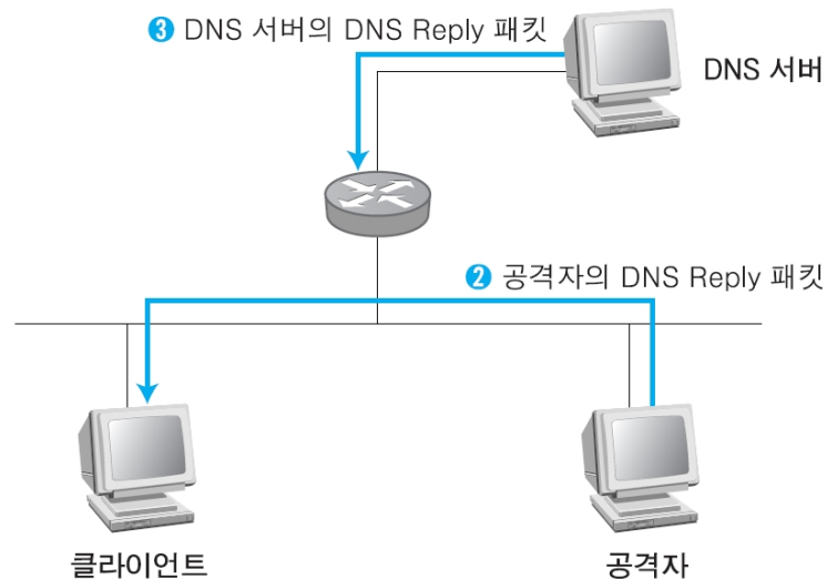
[그림 3-38] 공격자와 DNS 서버의 DNS Response
