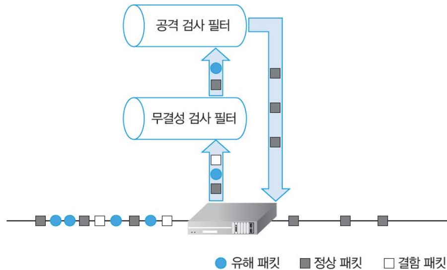
[그림 10-12] 침입 방지 시스템의 동작 원리
