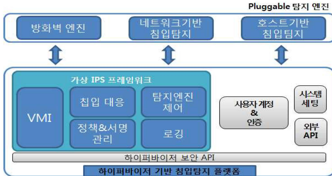
[ VMI 기반 침입탐지 시스템 (Xen 기반의 사례)]
