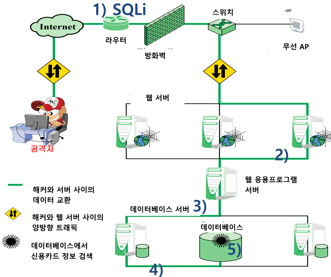
통상적 SQL 주입공격
