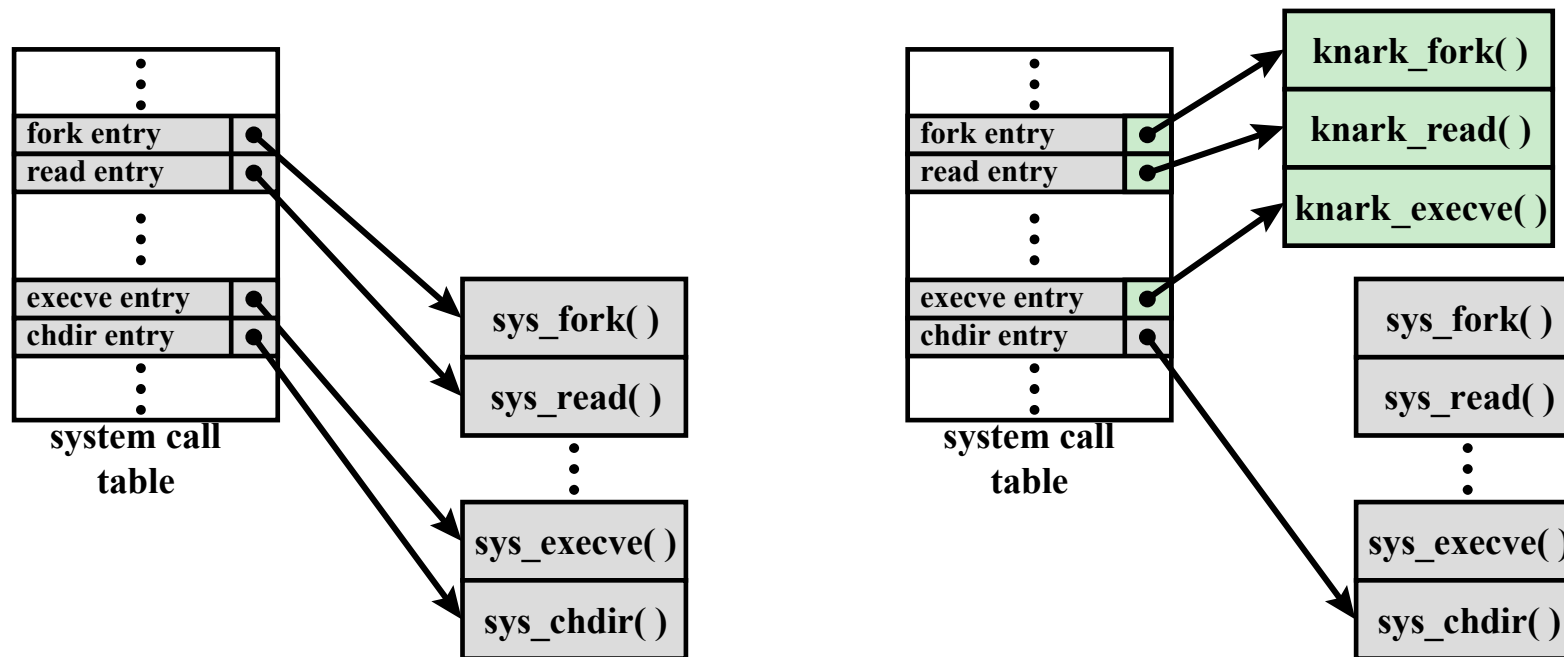
(a) 평범한 커널 메모리 계층
