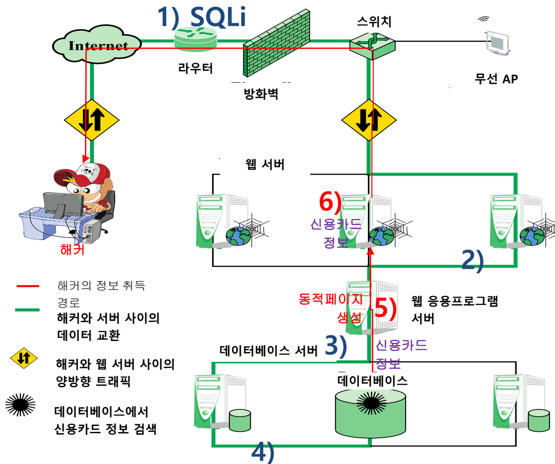
[ 전형적인 SQL 주입 공격 ]
