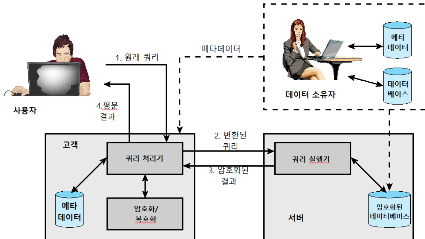
데이터베이스 암호화 기법
