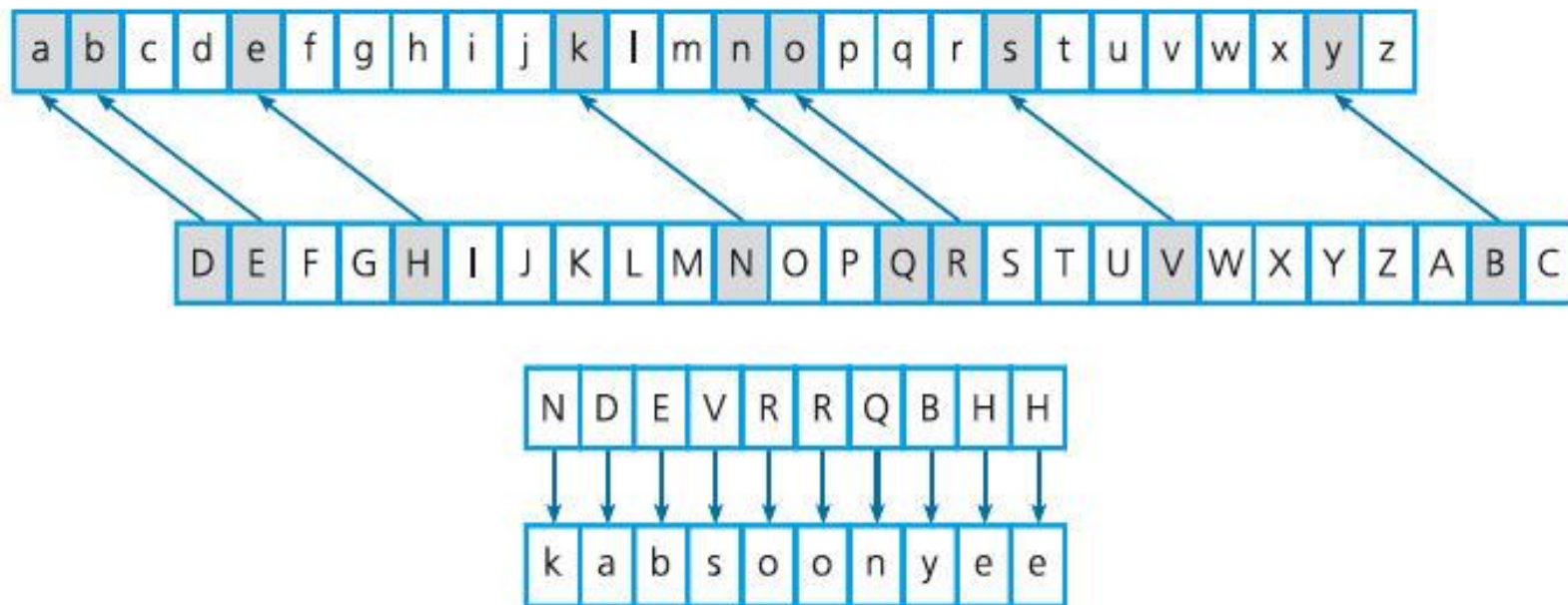
그림 3-4 · 암호문을 1문자씩 복호화하기
